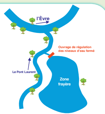
Frayère en eau durant toute la période de reproduction du brochet (mi-février à mi-mai)
